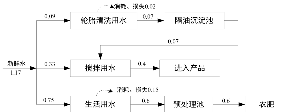
图 2-1 本项目水平衡图 ( \text{m}^3/\text{d} )
