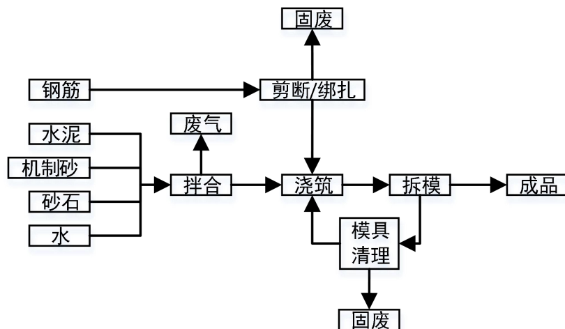
图 2-2 项目工艺流程及产污节点图
