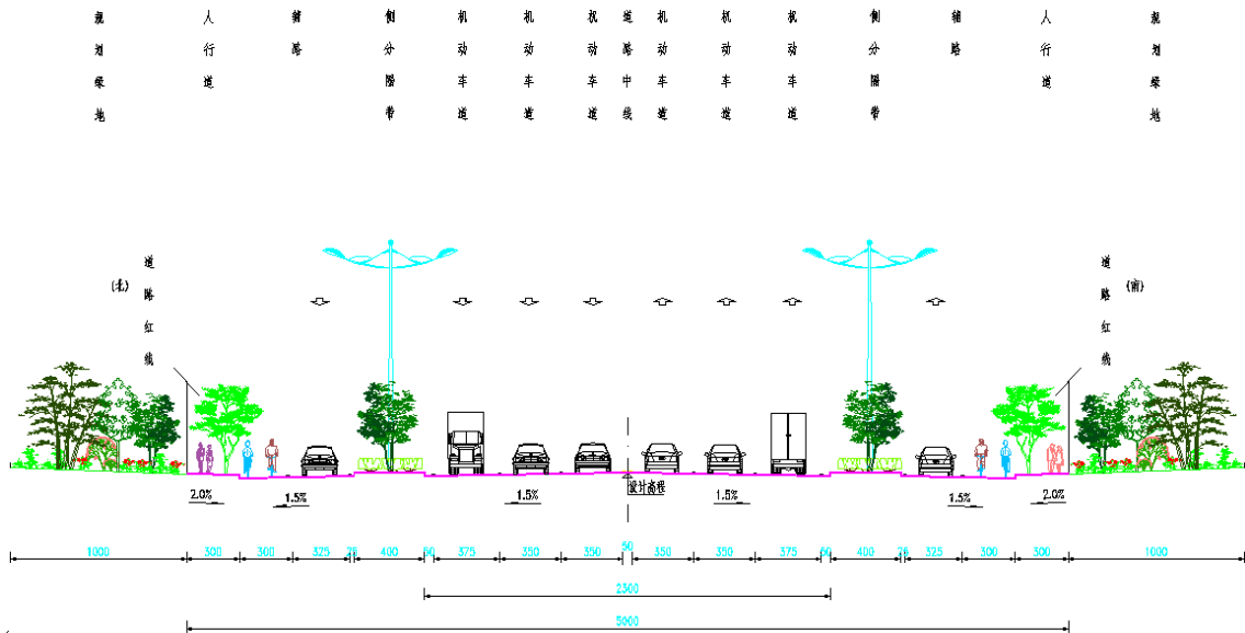
图 4-1 本项目 50m 道路横断面
