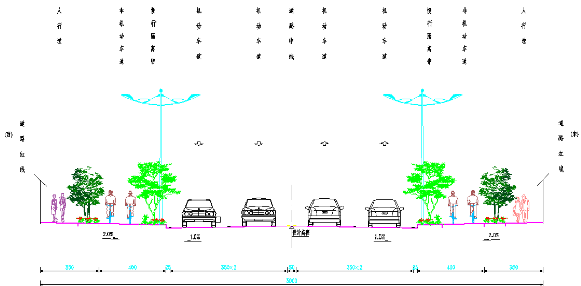
图 4-1 本项目 50m 道路横断面
