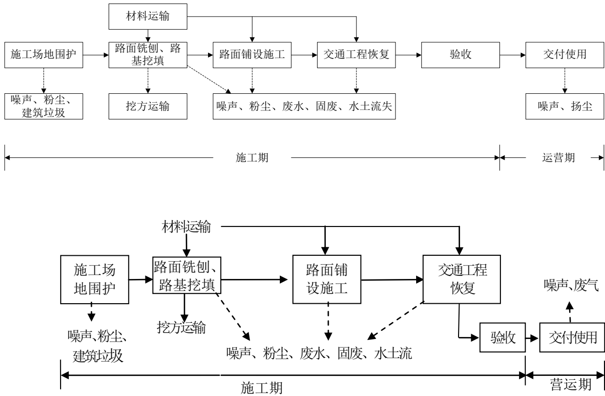
图4-1 项目工艺流程及产污环节图
